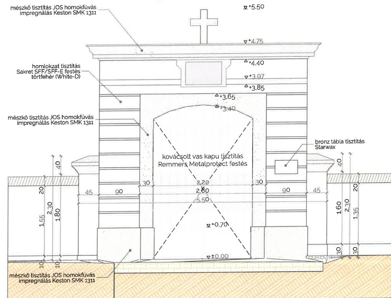
külső nézet
