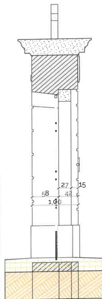
metszet
