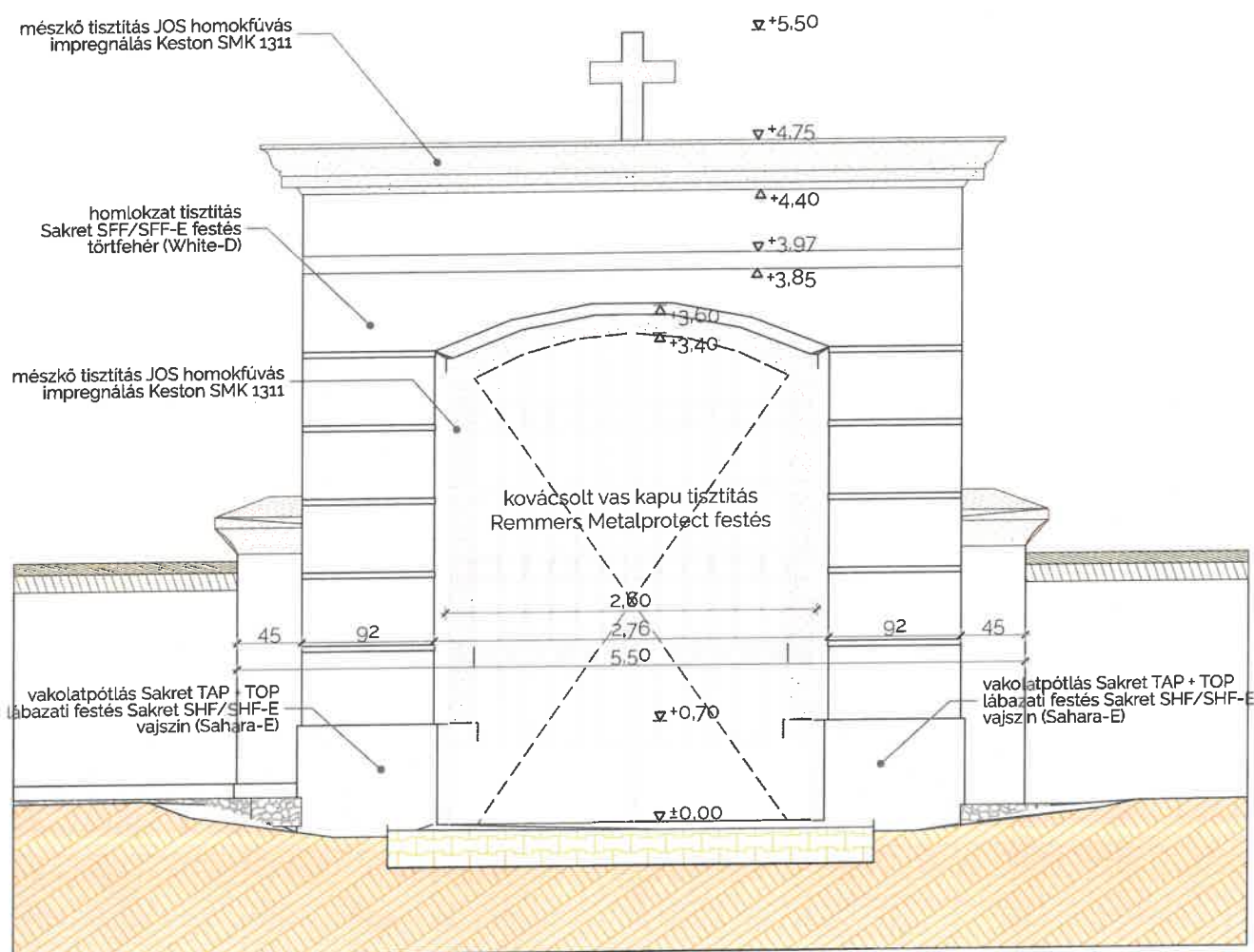
belső nézet
