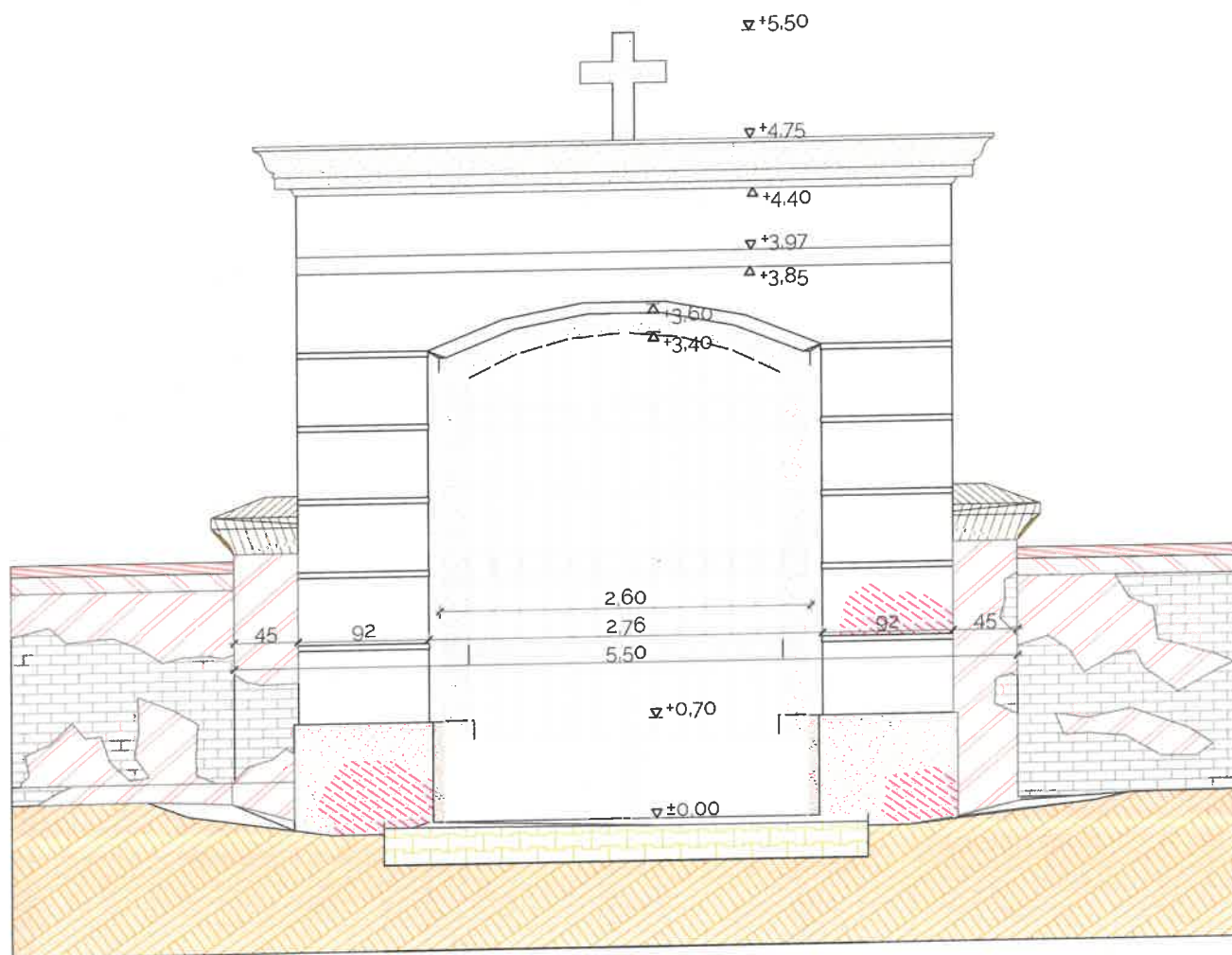
belső nézet
