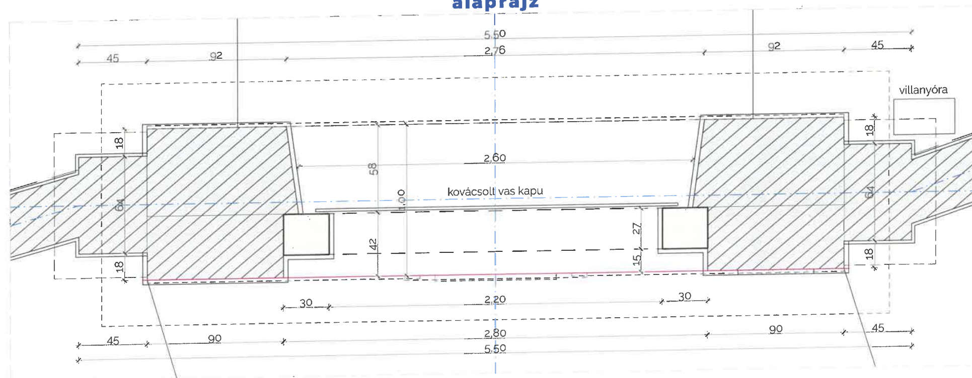
alaprész
