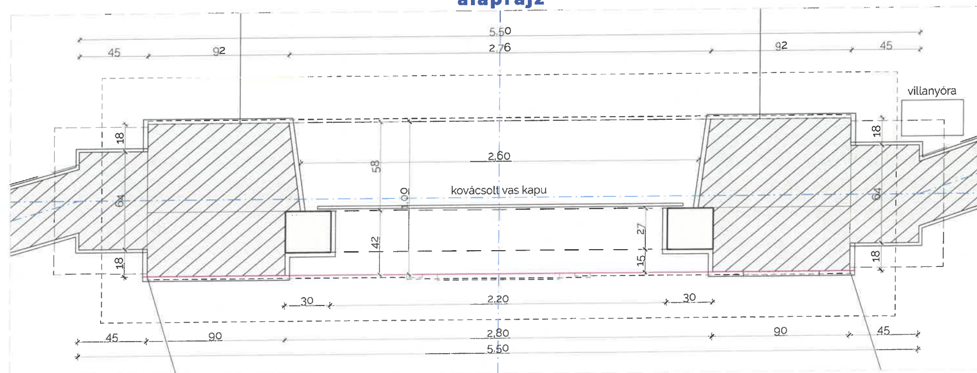
alaprajz
