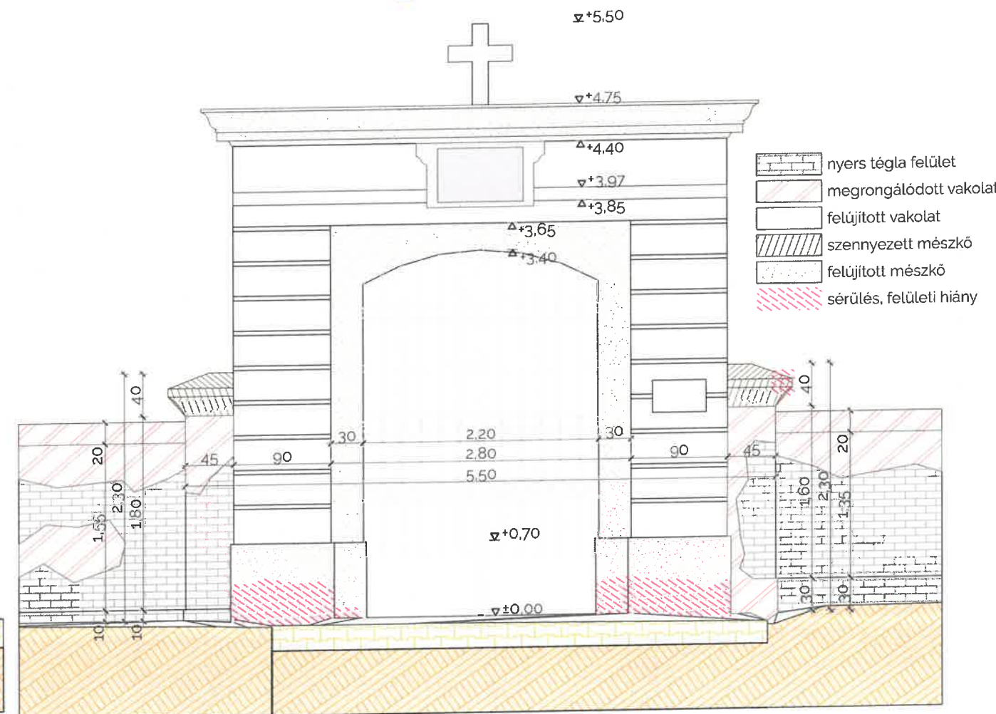
külső nézet
