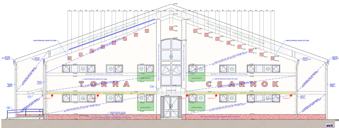
A nagyecenki tornacsarnok tervezett déli homlokzata (tervező: Molnár Attila Aladár)
